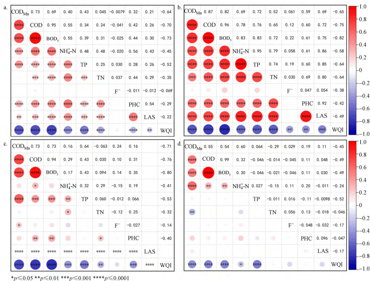
图5 主要水质因子与WQI的皮尔逊相关性分析(a.整体相关性,b.枯水期相关性,c.平水期相关性,d.丰水期相关性)
