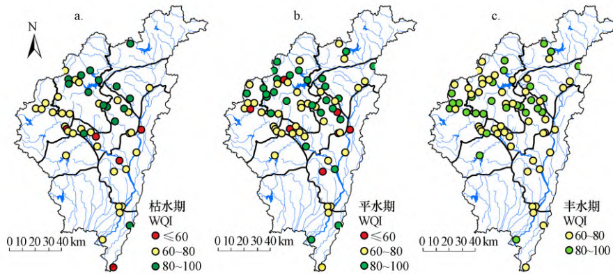
图3 不同水文期WQI空间分布(a.枯水期,b.平水期,c.丰水期)
