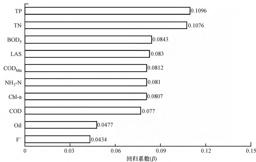
图2 LASSO回归模型中纳入指标的回归系数( \beta )排序
