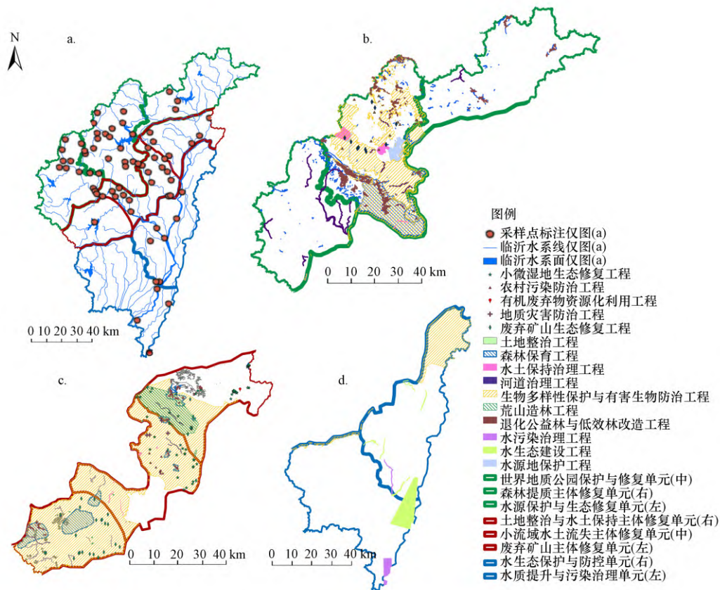
图1 研究区水质采样点(a)与治理工程分布(b.水源涵养生态修复区,c.水土保持生态修复区,d.水安全水生态修复区)
