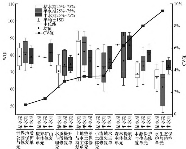
图4 8个生态修复单元在3个水期下的WQI表现与变异系数CV
